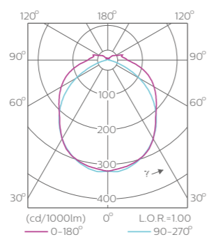
WT980 LEDtube Exd 1xLEDtube
